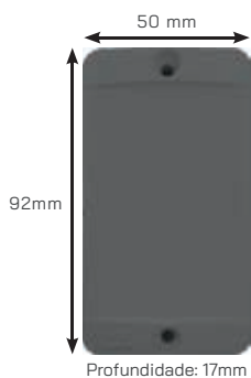
LPC4200 Placa para Condutele Cega
