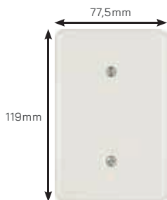
4x2 BE4200 Placa 4x2 Cega
